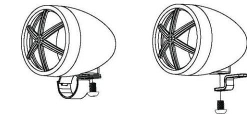
Схема монтажа колонок
